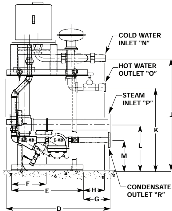
END ELEVATION
