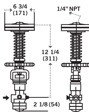
TYPE F15 PILOT 15 LBS (6.8 KG)
