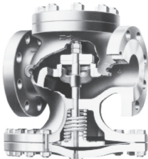
TYPE E8 MAIN VALVE
