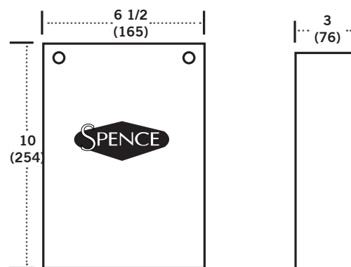
TYPE D208 ELECTRONIC TIME CONTROLLER (ETC)
