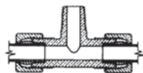
7B TEE
